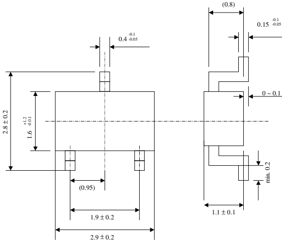
SOT-23 :
