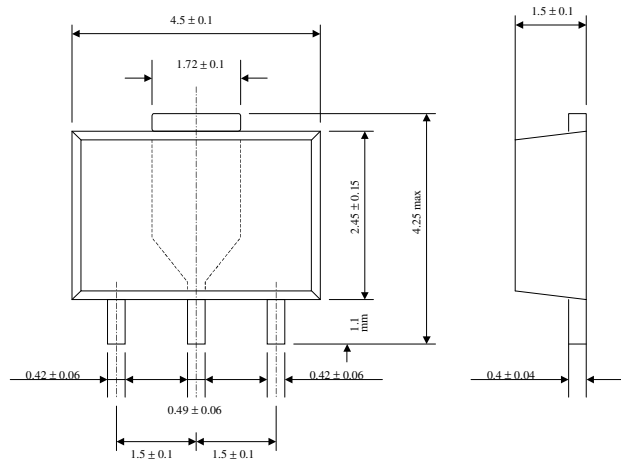
SOT-89 :
