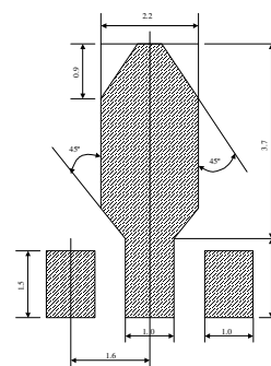
SOT-89
